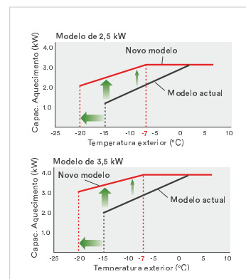
Maior potência no aquecimento.
