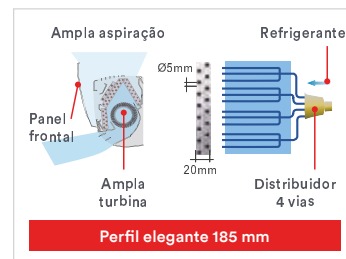
Novo design compacto e elegante.
